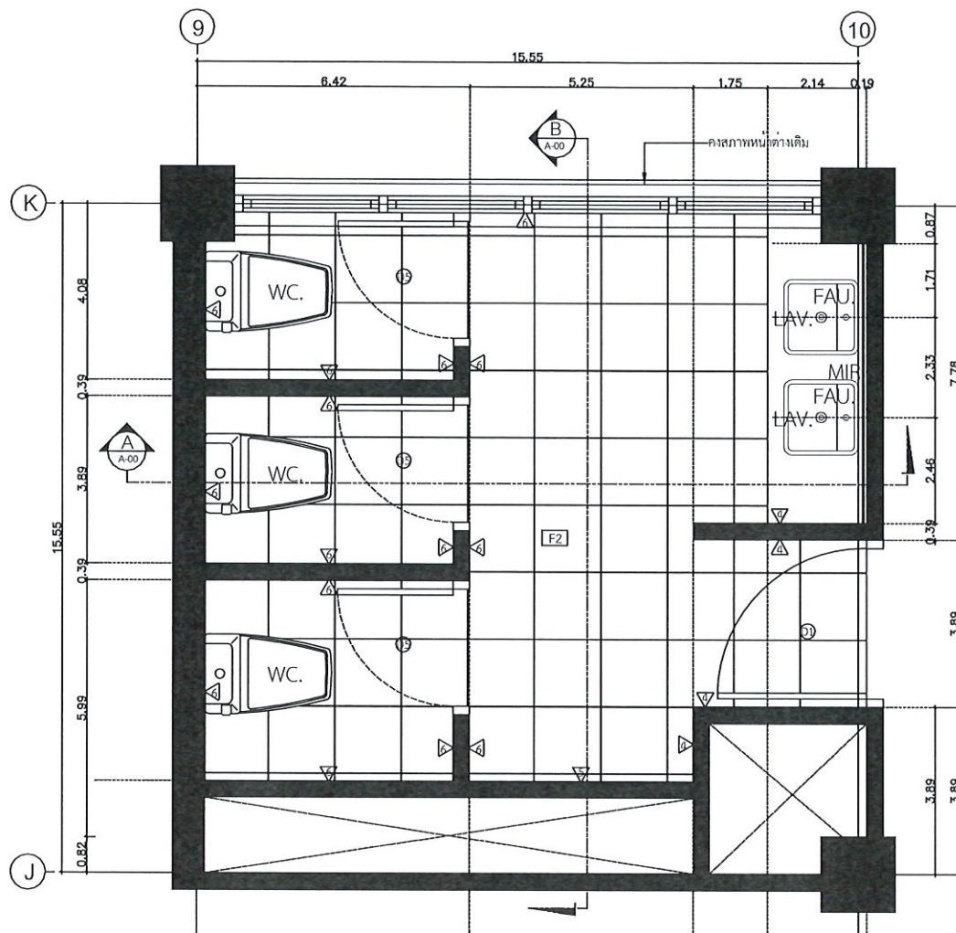
แปลนขยายห้องน้ำหญิงชั้น 2 มาตราส่วน 1:25
