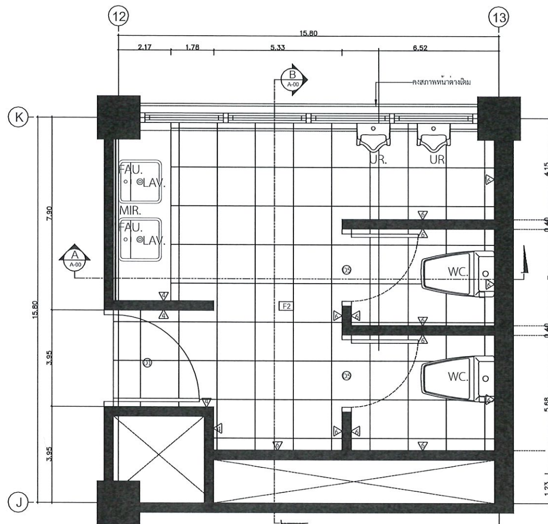
แปลนขยายห้องน้ำชายชั้น 2
