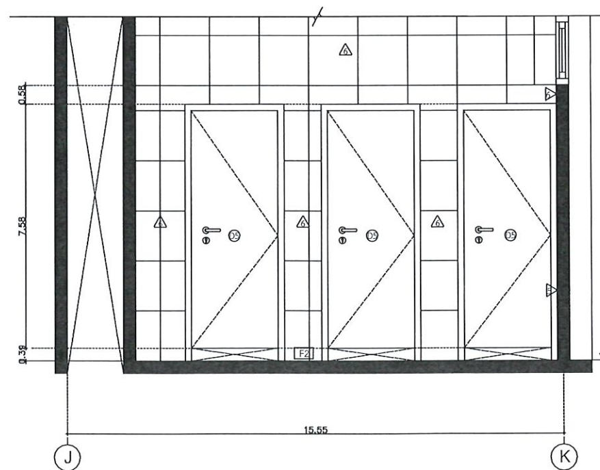
รูปตัด B-B ขยายห้องน้ำหญิงชั้น 2 มาตราส่วน 1:25
