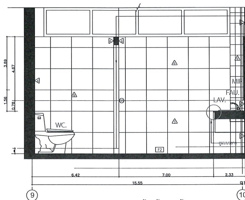
รูปตัด A-A ขยายห้องน้ำหญิงชั้น 2 มาตราส่วน 1:25
