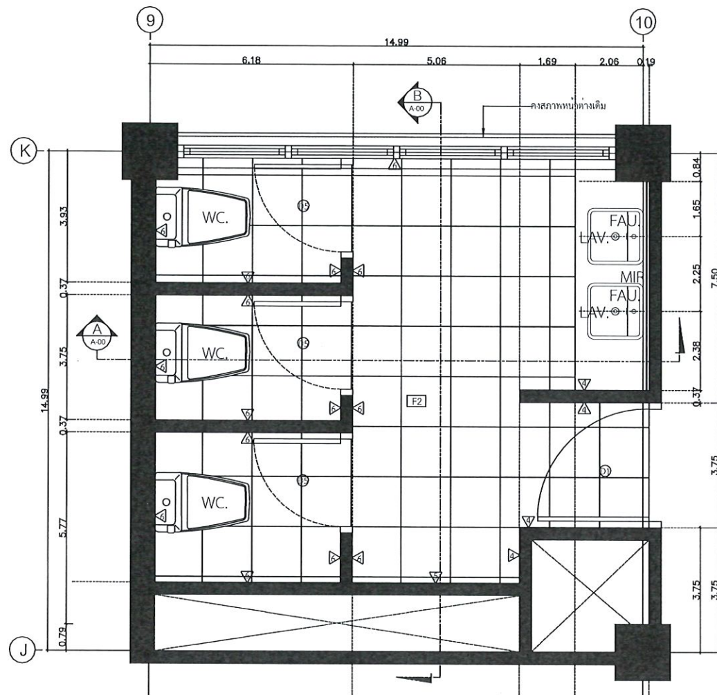
แปลนขยายห้องน้ำหญิงชั้น 3
