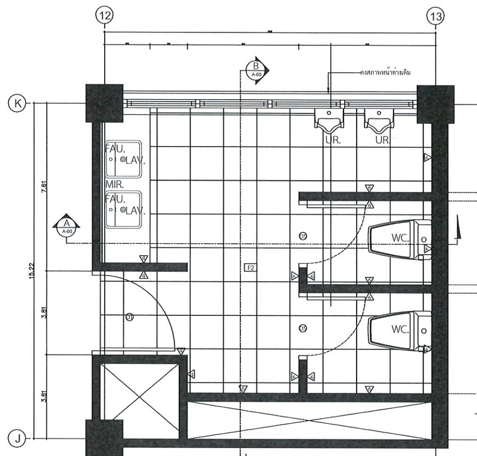
แปลนขยายห้องน้ำชายชั้น 3
